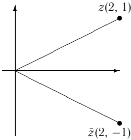
Рис. 25. Операция сопряжения
