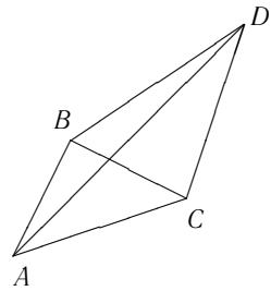
Рис. 31. Теорема Птолемея
