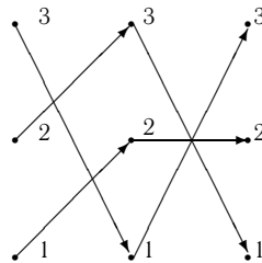
Рис. 13. Умножение подстановок
