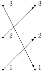
Рис. 12. Граф подстановки
