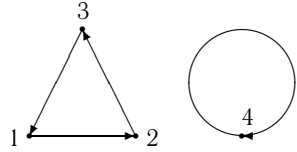
Рис. 16. Граф перестановки
